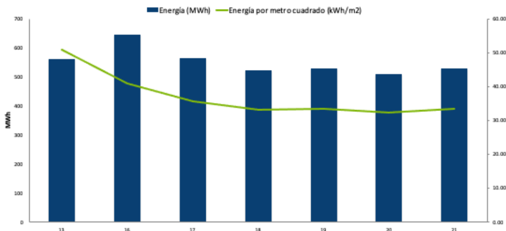
Gráfica 17. Relación del consumo de energía por metro cuadrado de los años 2013 a 2021.
